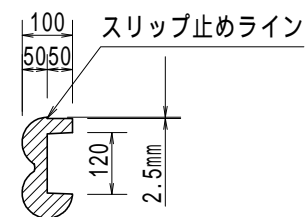
A-A断面図
