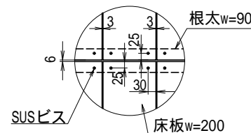
デッキ板継目部
