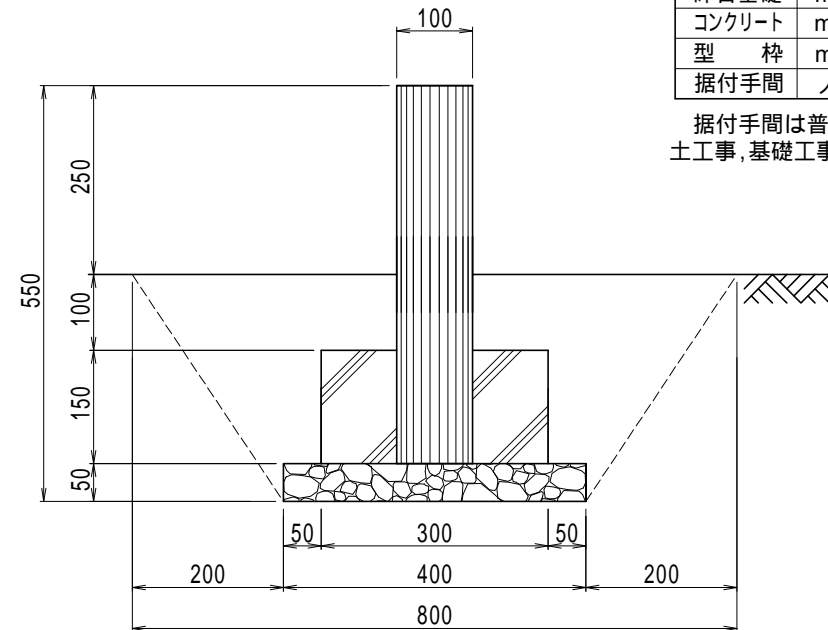
標準基礎図S=1:10
