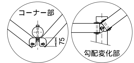
三次元継手金具詳細図
