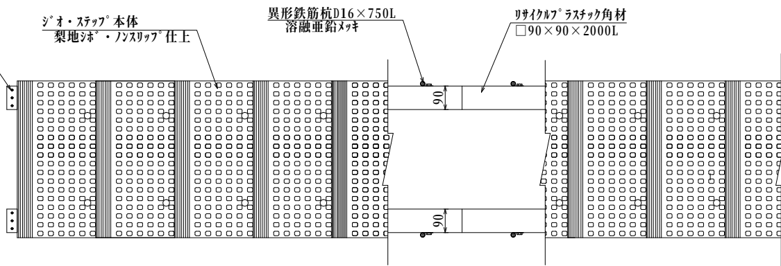
平面図S=1：10
