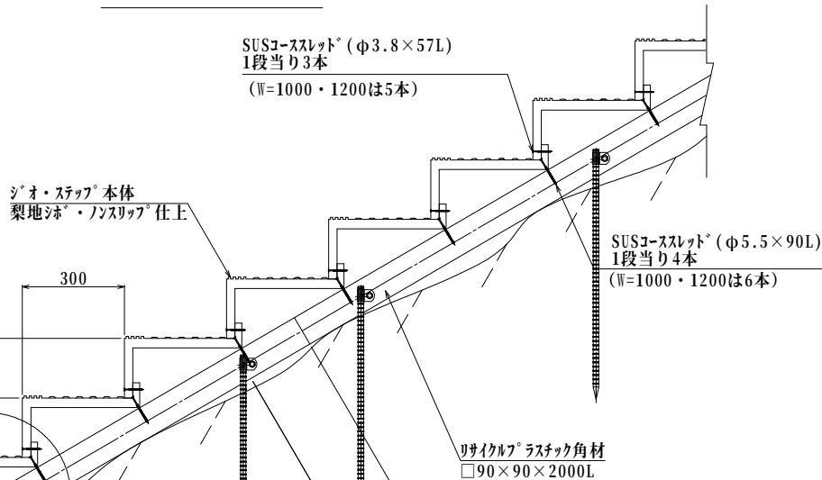
側面図S=1：10
